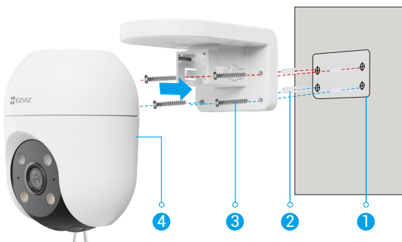
Fig. 2 Montage mural
