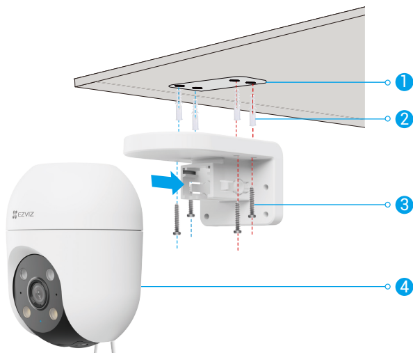
Fig. 1 Montage au plafond
